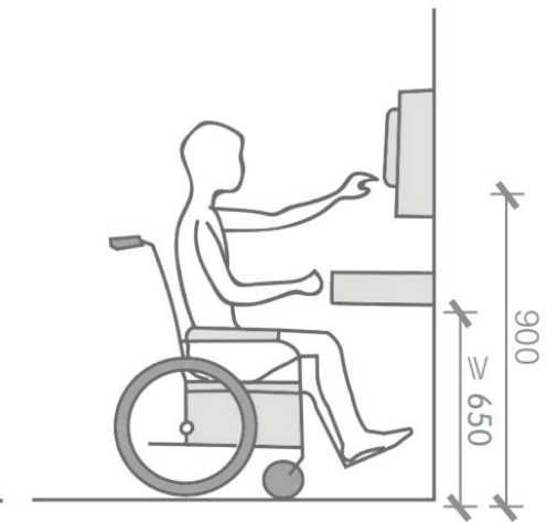
图：低位电话
