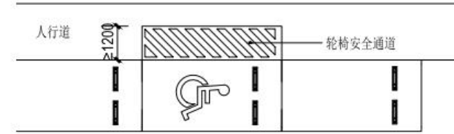
无障碍停车位示意图-1(mm)
