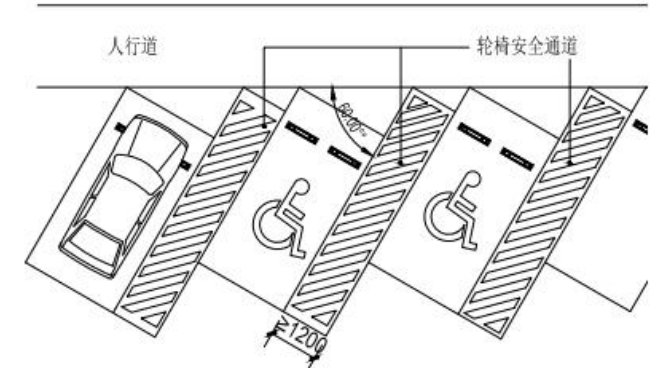
无障碍停车位示意图-3(mm)
