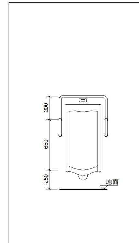
小便池正立面图
