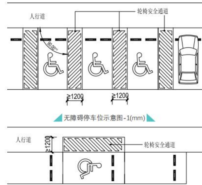
无障碍停车位示意图-2(mm)
