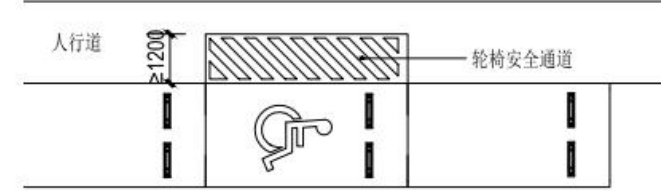
无障碍停车位示意图-2(mm)
