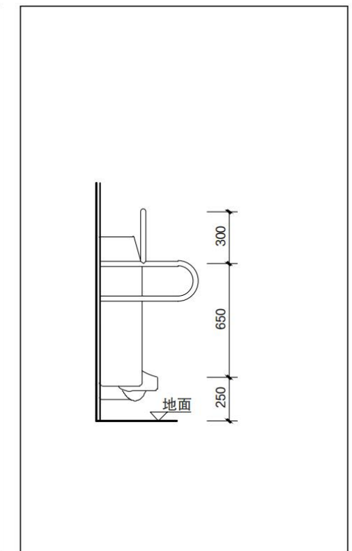
小便池侧立面图
