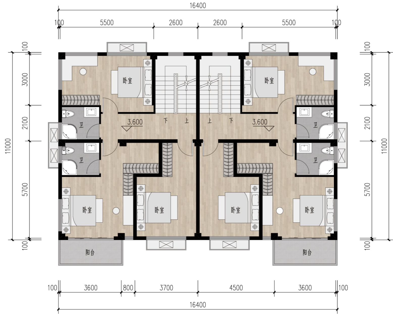
二层平面图
