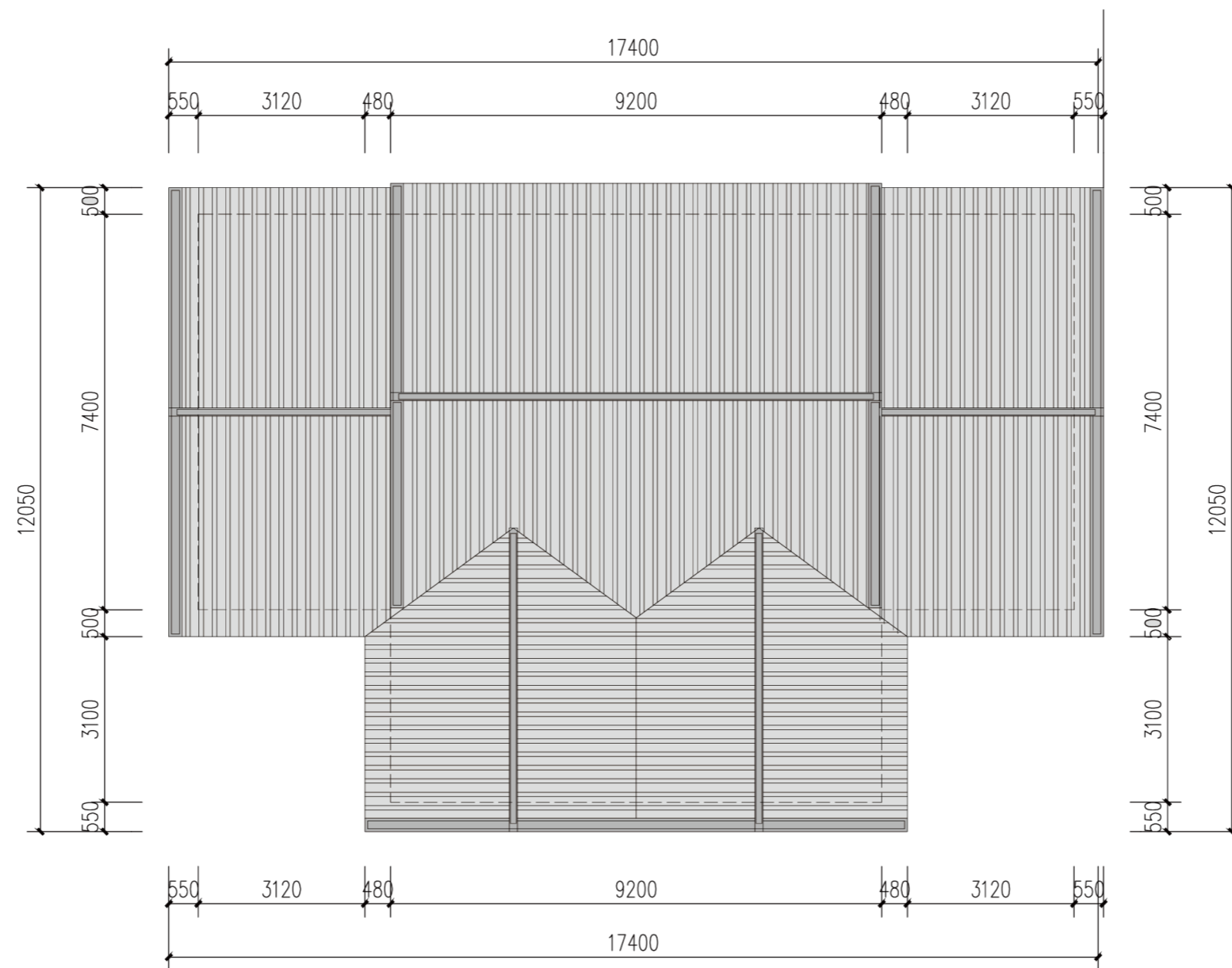
屋顶平面图
