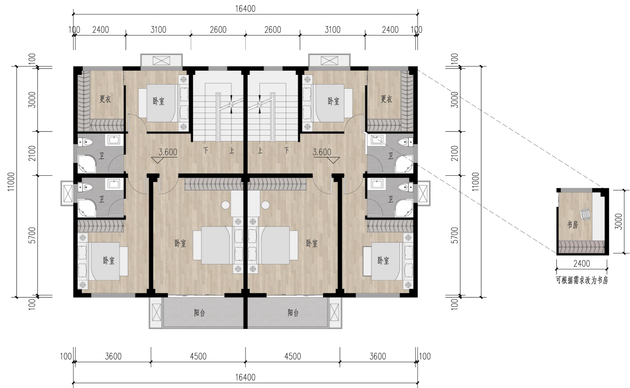
二层平面图
