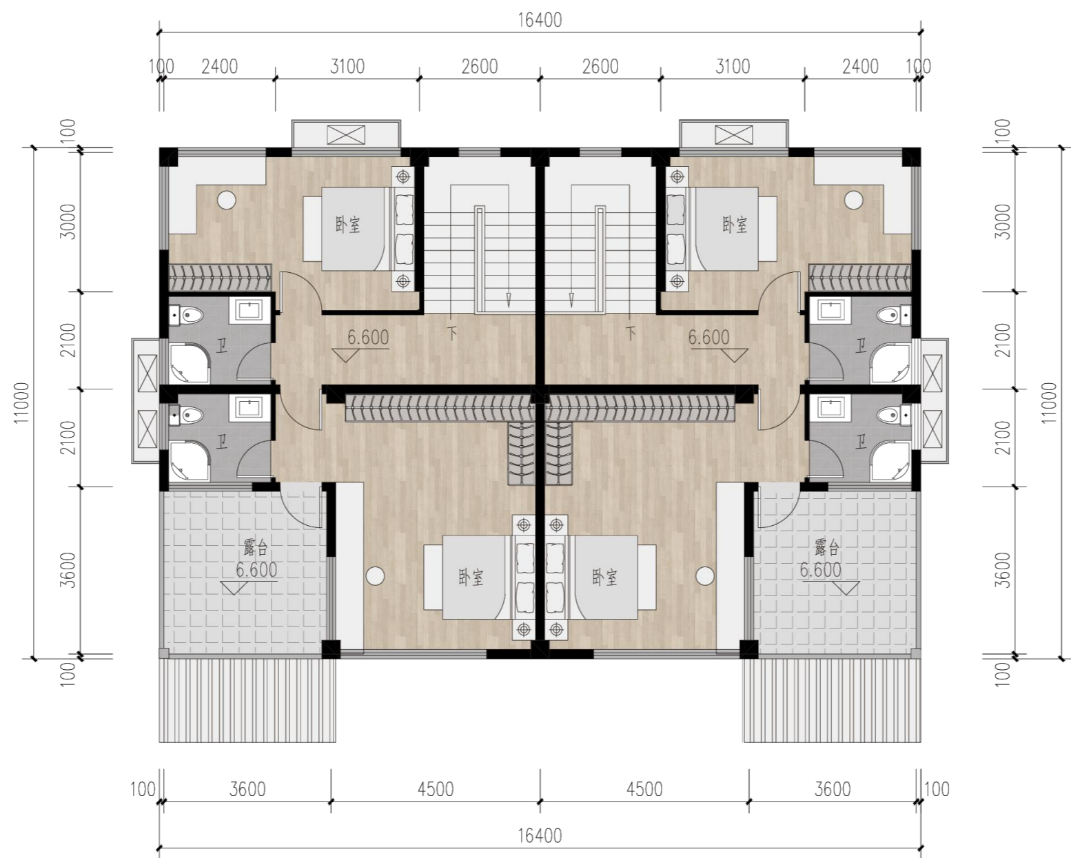
三层平面图
