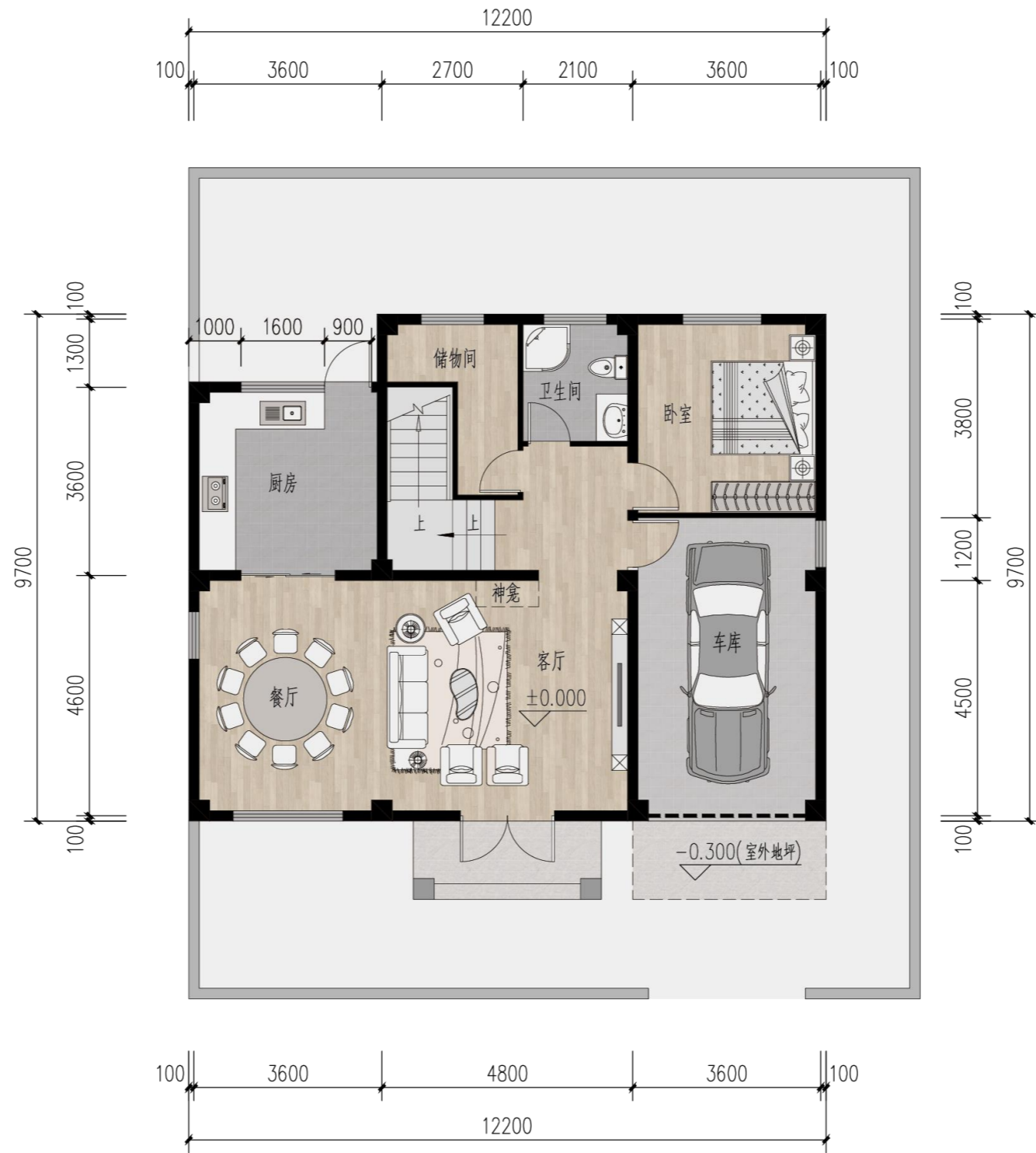
一层平面图
