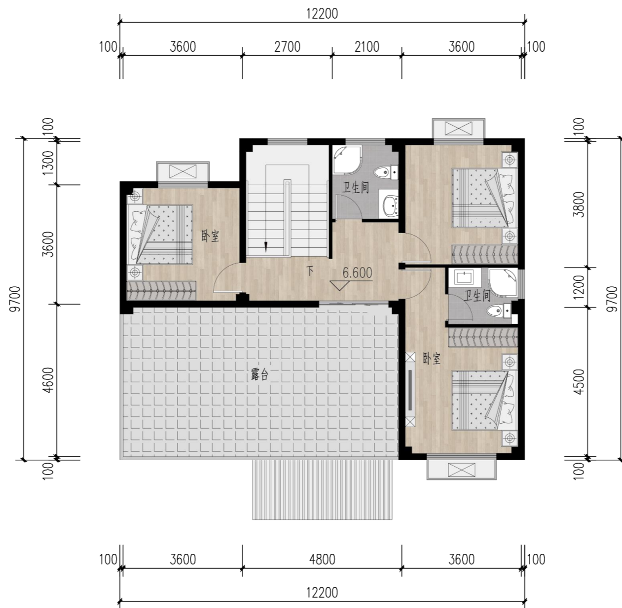
三层平面图
